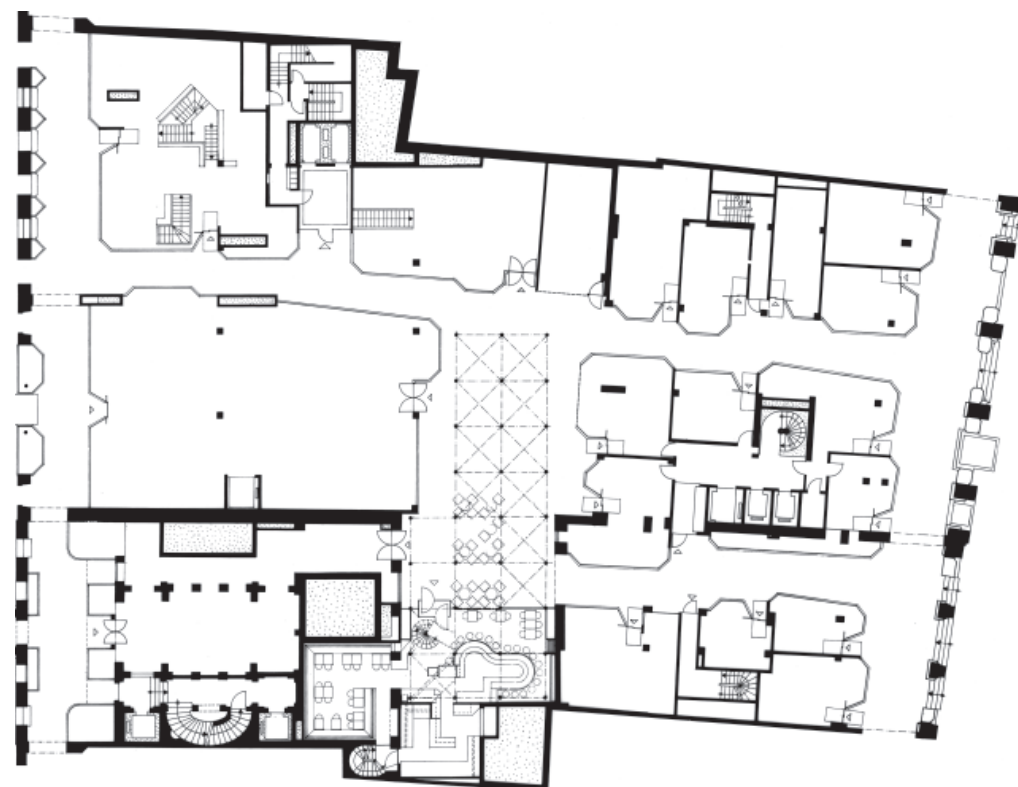
rechts: Grundriss des Erdgeschosses mit Passagen, Restaurant und Läden oben: Axometrie des Restaurants rechts: das zweigeschossige Restaurant unten rechts: die Bar im Restaurant
